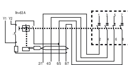
DDA 204
