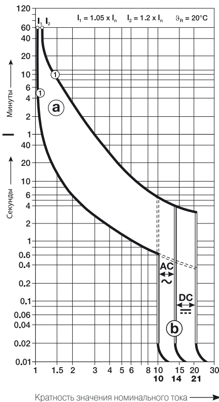
Характеристика K
