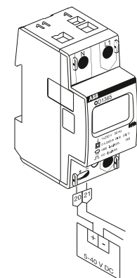
Импульсный выход
