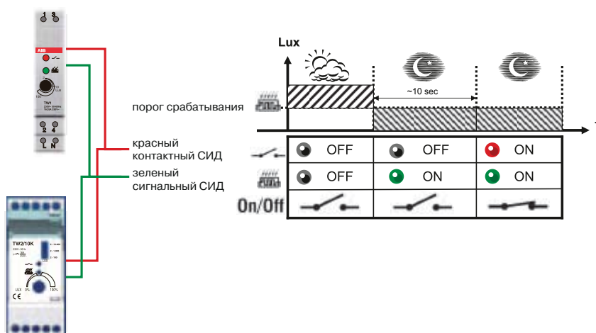
ТW1 и ТW2/10K принцип работы
