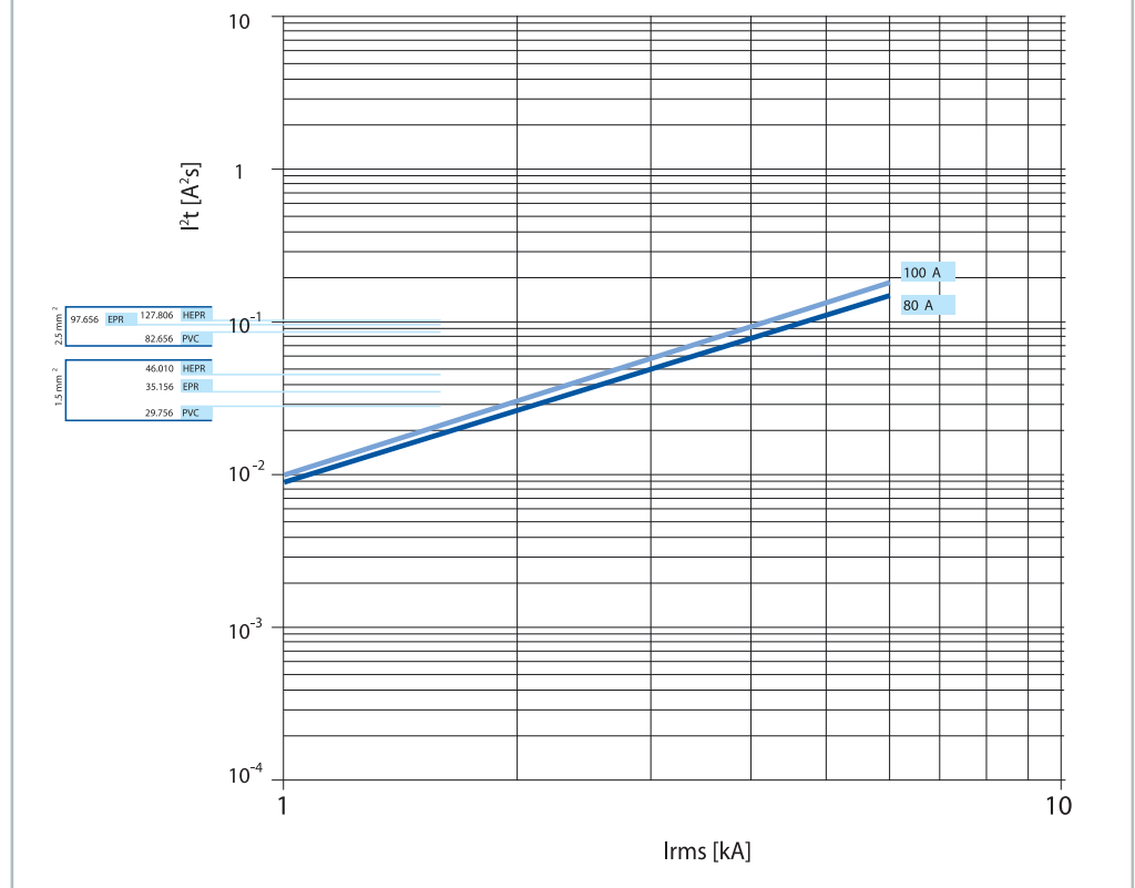
S 280 80-100 A, характеристика B
