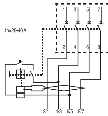
DDA 204
