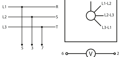
MCV4
