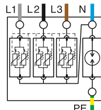
OVR T2 3N 40 275s P OVR T2 3N 70 275s P OVR T1+2 3N 7 275s P
