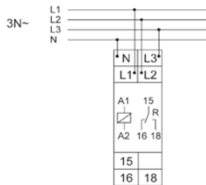
Подключение E 236-US 1.1D
