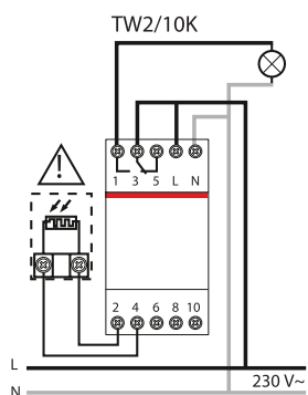
ТW1 и ТW2/10K принцип работы
