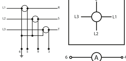
MCA4
