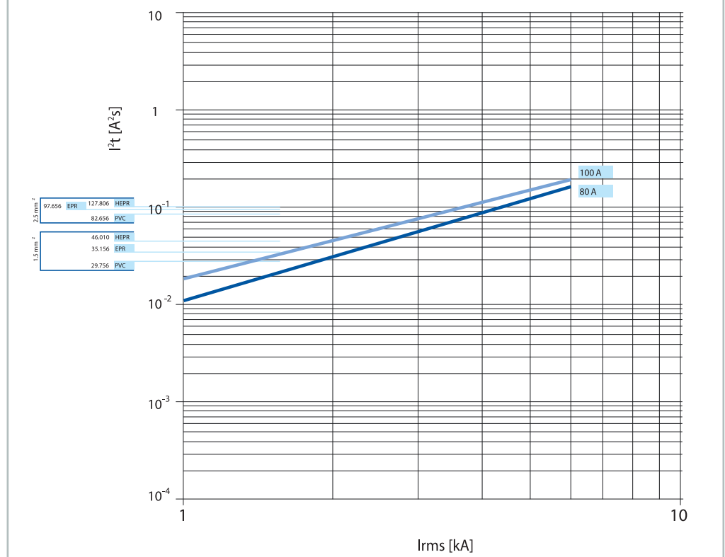
S 280 80-100 A, характеристика C
