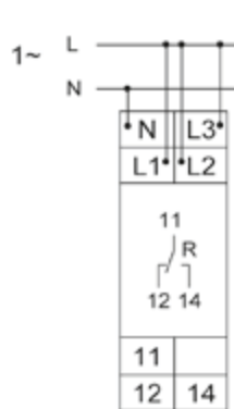
Диаграмма работы E 236-US 1.1 и US 2.1
