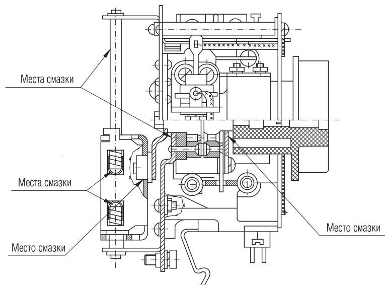
Рисунок А.13 - Места смазки электромагнитного привода.
