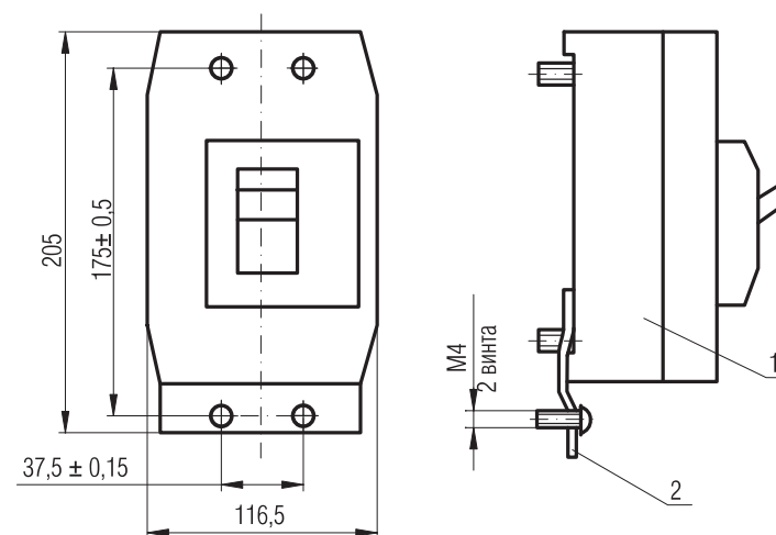
1 - выключатель; 2 - скоба.
