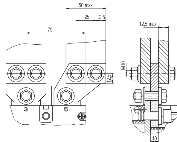
Рисунок В.6 - Переднее присоединение шиной или двумя шинами «плашмя» с переходником или кабелями (1-4) с кабельным наконечником ГОСТ 7387-82, ГОСТ 7386-80, с контактным стержнем \Phi 10 мм для выключателей типа ВА08-040Х, ВА08-063Х, ВА08-080Х (остальное см. рисунок А.1, А.2)
