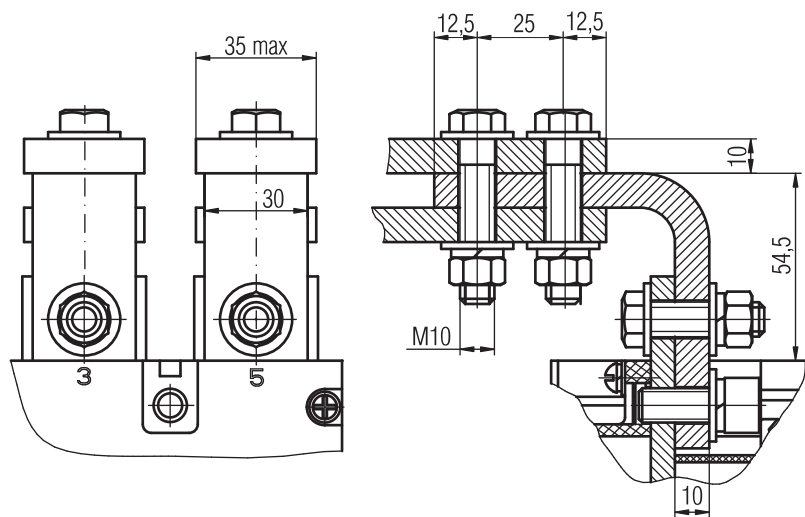
Рисунок В.14 - Заднее присоединение шиной или двумя шинами, кабелями с кабельными наконечниками для выключателей типа ВА08-040Х, ВА08-063Х, ВА08-080Х (остальное см. рисунок А.1, А.2)
