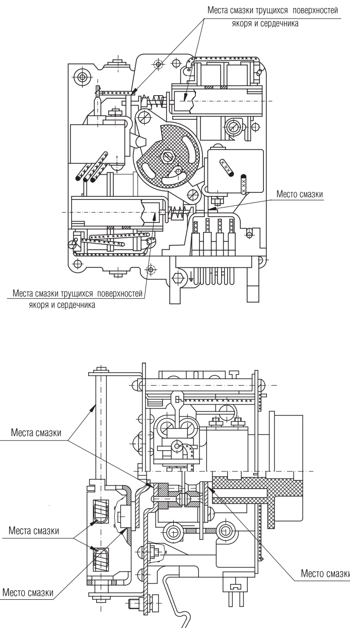
Рисунок Г.15 - Места смазки электромагнитного привода
