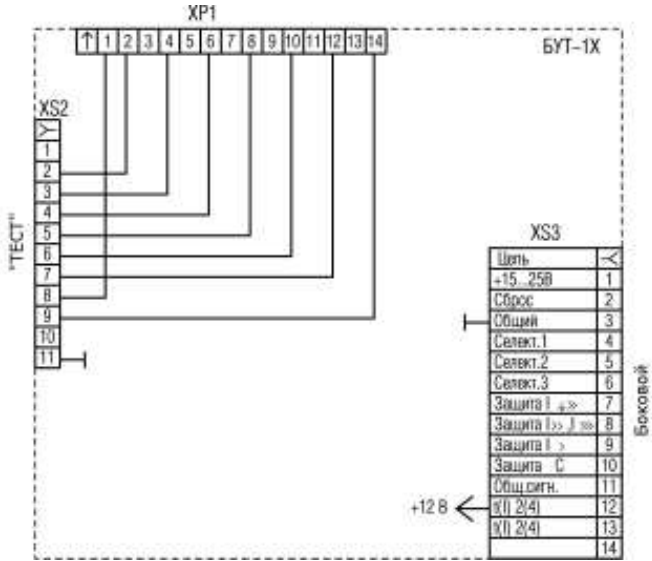
Рисунок Д. 18- Схема разъемов блока БУТ-1Х (к роме БУТ-14)
