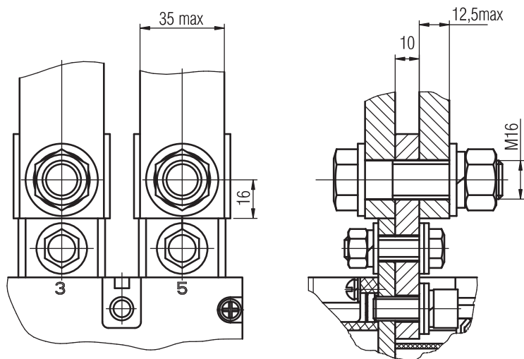
Рисунок В.7 - Переднее присоединение шиной или двумя шинами, кабелем или двумя кабелями с кабельными наконечниками ГОСТ 7386- 80 с контактным стержнем \Phi 16 мм для выключателей типа ВА08-040Х, ВА08-063Х, ВА08-080Х (остальное см. рисунок А.1, А.2)
