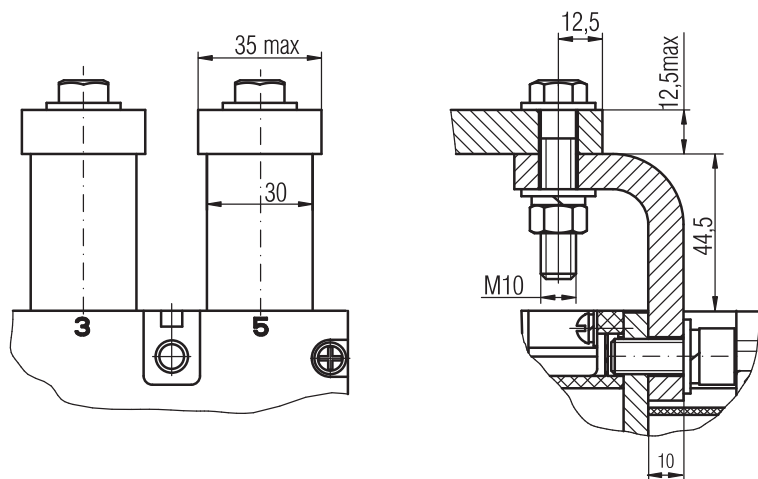
Рисунок В.13 - Заднее присоединение шиной или двумя шинами, кабелями с кабельными наконечниками для выключателей типа ВА08-040Х, ВА08-063Х (остальное см. рисунок А.1)
