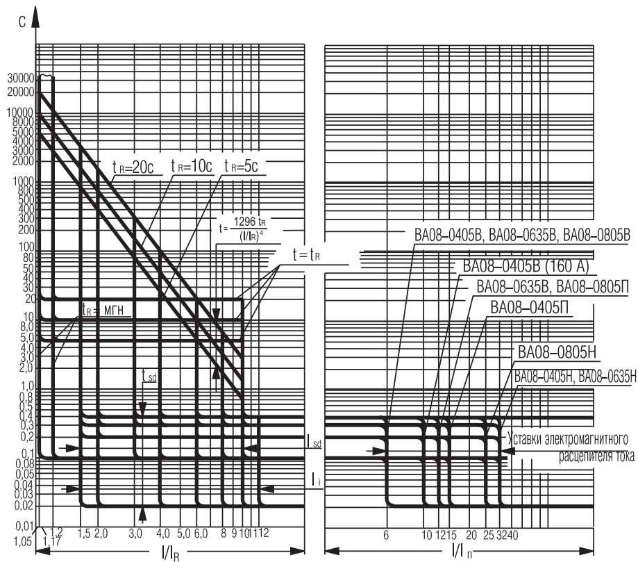
Рисунок Е.8 - В время-токовая характеристика выключателя переменного тока с электронным (микропроцессорным) расцепителем тока и электромагнитным расцепителем тока
