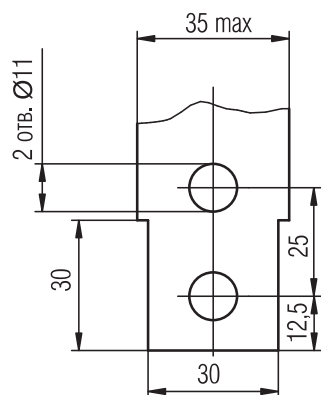
Рисунок В.2 - Переднее присоединение шиной «плашмя» для выключателей типа ВА08-040Х, ВА08-063Х, ВА08-080Х (остальное см. рисунок А.1, А.2)
