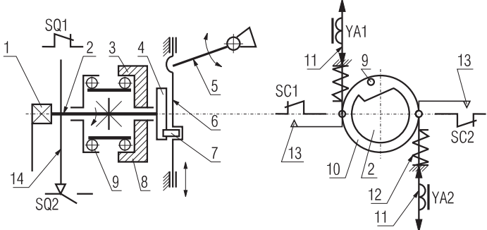
1-ручка; 2-валик; 3-кольцо неподвижное; 4-эксцентрик; 5-рукоятка; 6-каретка; 7-ролик; 8-ролики стопорные; 9-ролики ведущие; 10-кольцо подвижное; 11-якоря; 12-пружины; 13-упоры; 14-пластина
