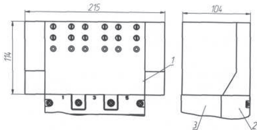
1 - козырек; 2 - крышка выключателя; 3 - корпус выключателя;
