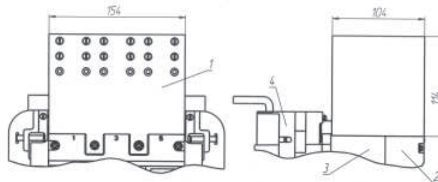
1 - козырек; 2 - крышка выключателя; 3 - корпус выключателя; 4 - основание Рисунок Г.18 а - Козырек выключателя, устанавливаемый , устанавливаемый на выключатели выдвижного исполнения
