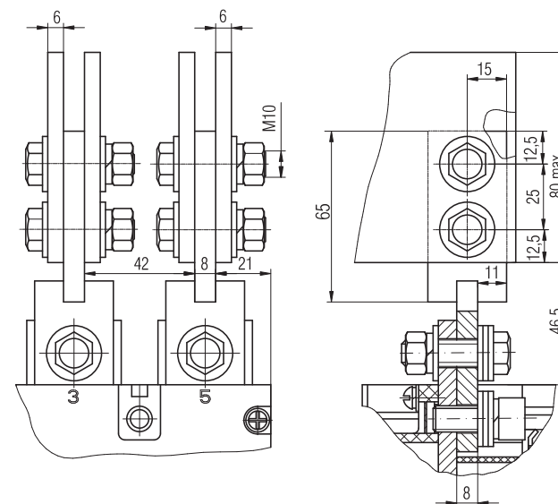
Рисунок В.11 - Присоединение шиной или двумя шинами на «ребро»или кабелями с кабельным неконечником для выключателей типа ВА08- 040Х, ВА08- 063Х для переднего и заднего присоединения (остальное см.рисунок А.1).
