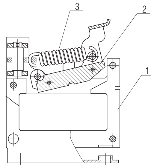
1 - сердечник; 2 - якорь; 3 - пружина Рисунок Г.3 - Электромагнитный расцепитель
