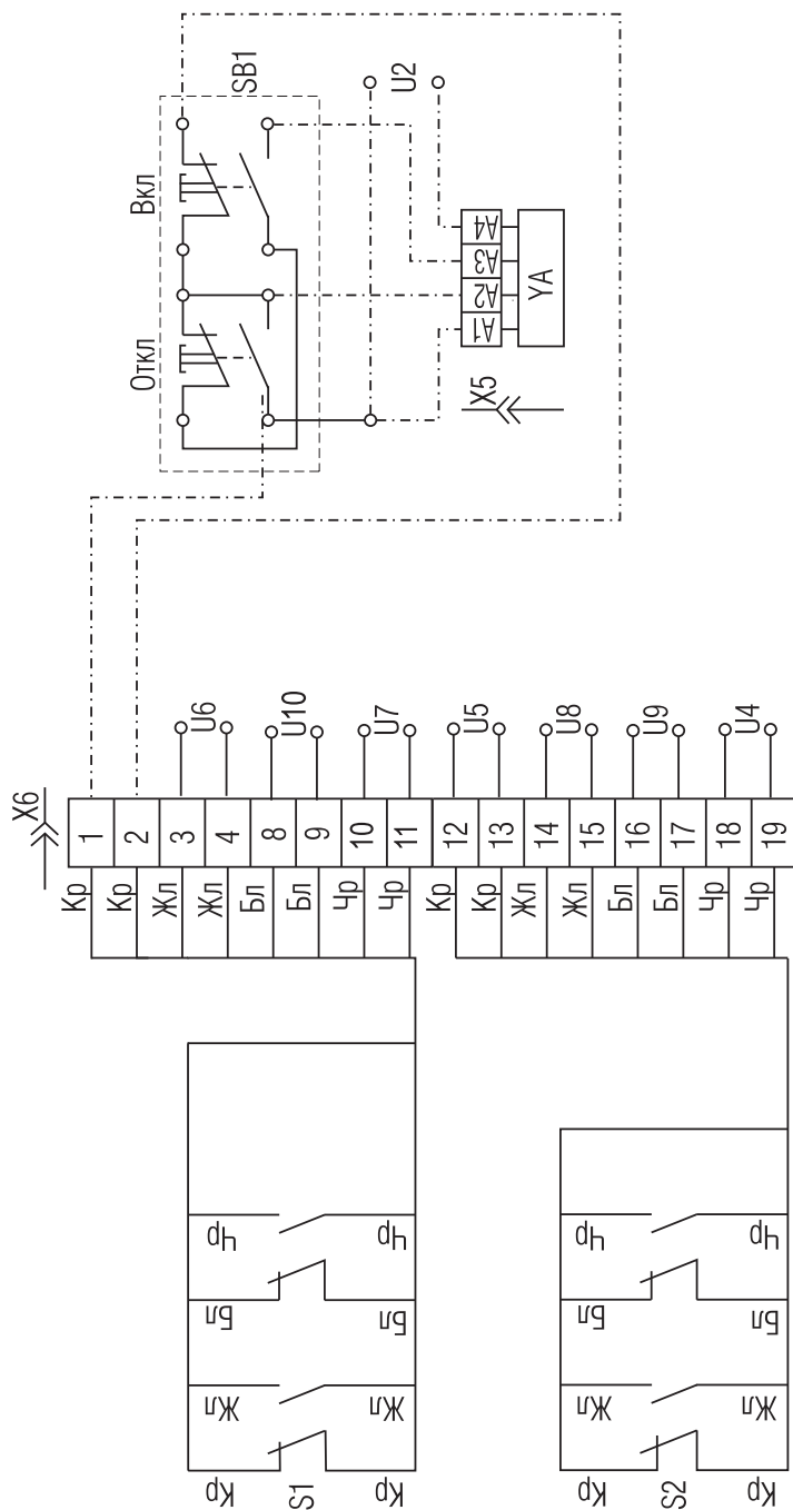
Рисунок Д.15 - Схема электрическая соединений дополнительных сборочных единиц выключателей выдвигного исполнения (ручной или электромагнитный привод, вспомогательные контакты, дополнительные вспомогательные контакты)
