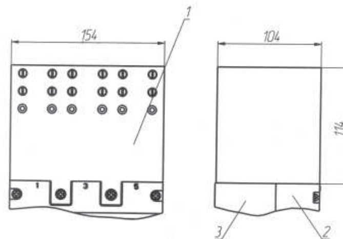
1 - козырек; 2 - крышка выключателя; 3 - корпус выключателя; Рисунок Г.18 - Козырек выключателя, устанавливаемый по рисункам приложения В, кроме рисунка В.6
