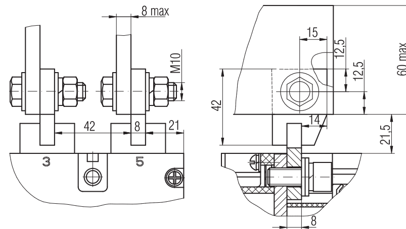
Рисунок В.11 - Присоединение шиной или двумя шинами на «ребро»или кабелями с кабельным неконечником для выключателей типа ВА08- 040Х, ВА08- 063Х для переднего и заднего присоединения (остальное см.рисунок А.1).
