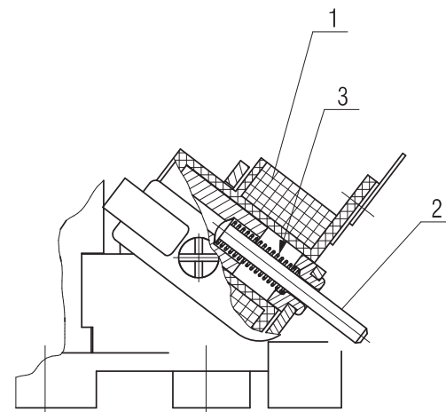
1 - катушка; 2 - шток; 3 - пружина Рисунок Г.4 - Расцепитель независимый
