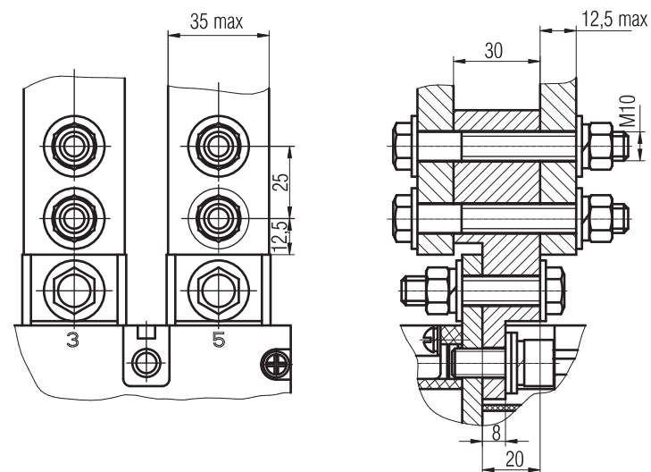
Рисунок В.5 - Переднее присоединение двумя шинами «плашмя» с переходником для выключателей типа ВА08- 080Х (остальное см. рисунок А.1, А.2)
