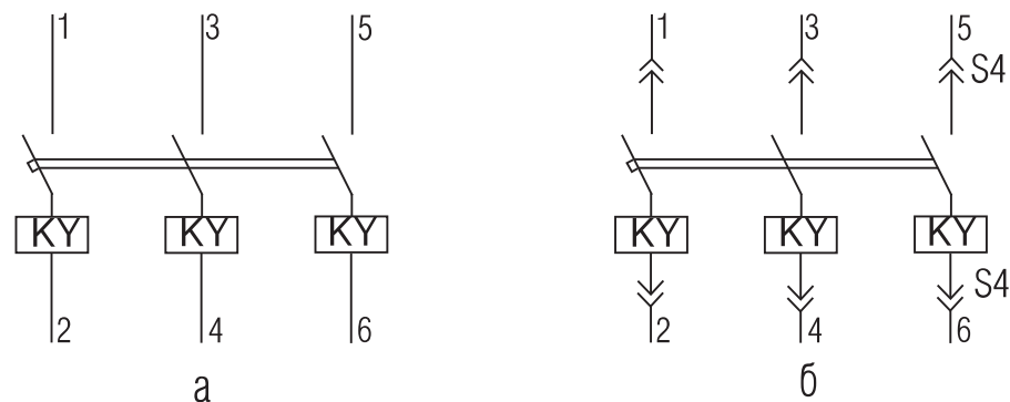
а- стационарное исполнение; б- выдвижное исполнение Рисунок Д.3 - Схема электрическая принципиальная выключателей с электромагнитными расцепителями
