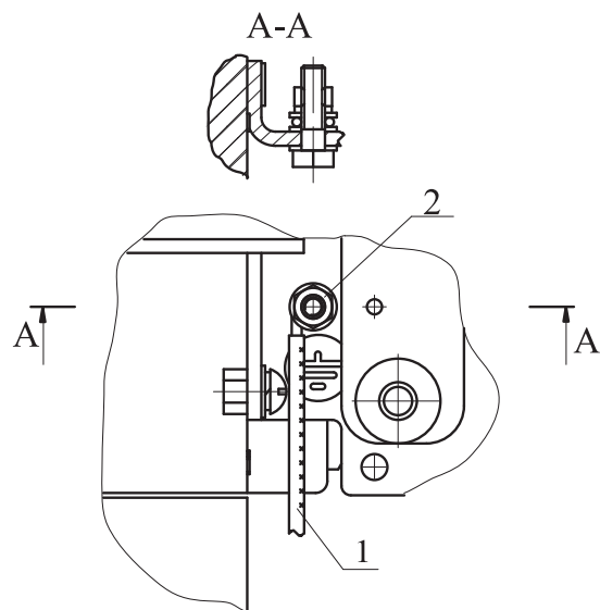
Рисунок Г.24 - Соединитель типа РПММ1-14
