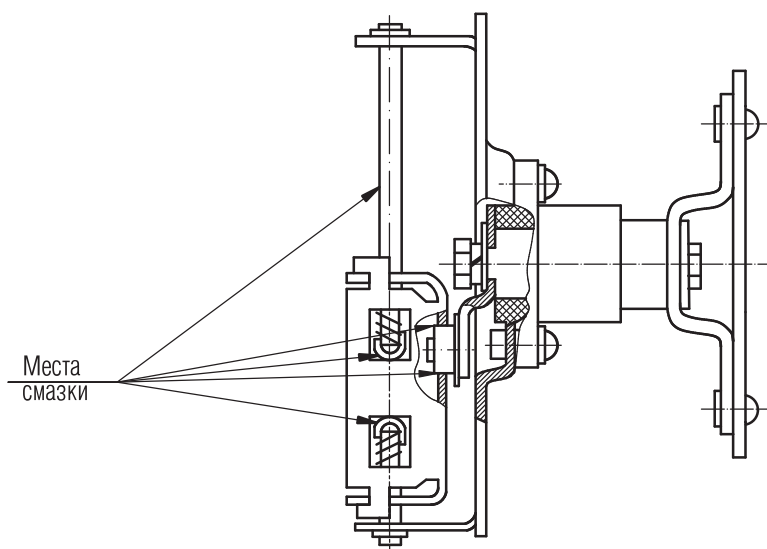
Рисунок Г.16- Места смазки ручного дистанционного привода выключателей выдвижного исполнения
