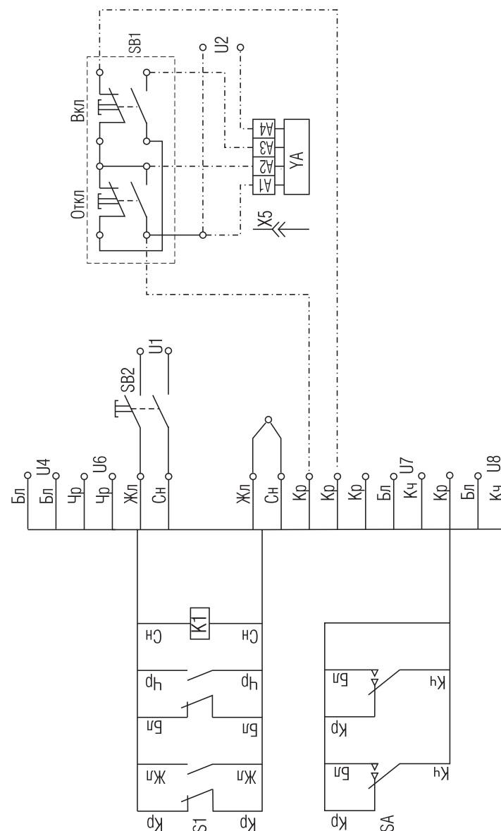
Рисунок Д.10 - Схема электрическая соединений дополнительных сборочных единиц выключателей стационарного исполнения (ручной или электромагнитный привод, вспомогательные контакты, микропереключатели)
