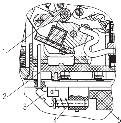
Рисунок Г.19- Блокировка перемещения выдвижной части при включенном выключателе
