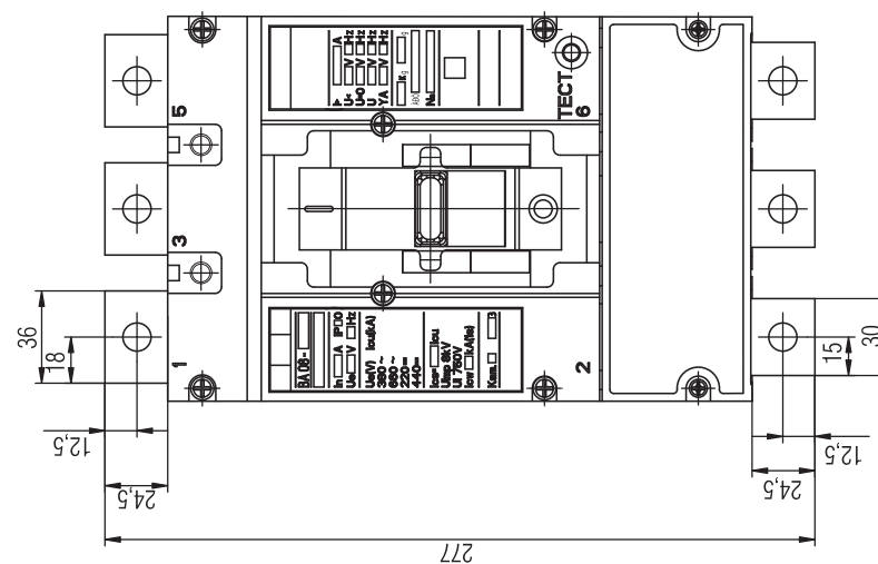
Рисунок А.2 - Выключатели типа ВА08-040Х, ВА08-063Х, ВА08-080Х стационарного исполнения на токи не более 800 А (остальное см. рисунок А.1)
