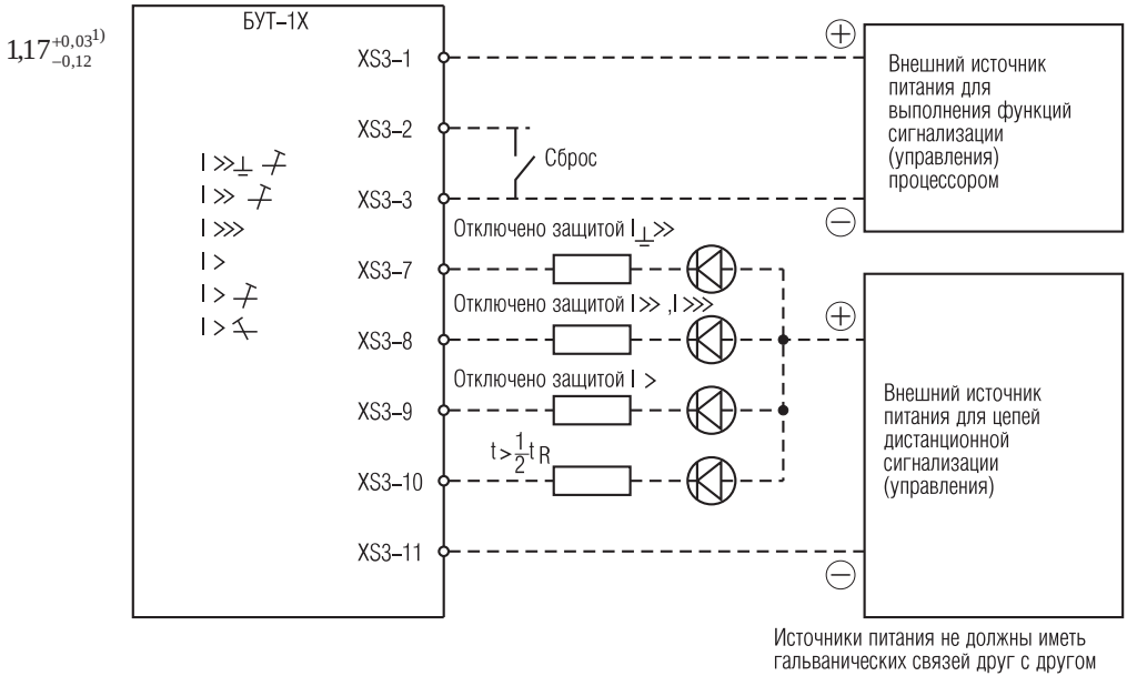
Рисунок Д. 19 - Схема подключения цепей сигнализации (управления)
