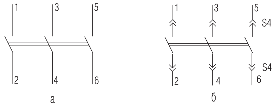
а- стационарное исполнение; б- выдвижное исполнение Рисунок Д.4 - Схема электрическая принципиальная выключателей без расцепителей тока
