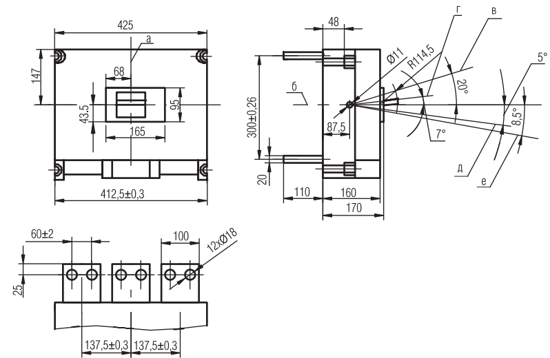
Масса - не более 49 кг; а - ось вертикальная; б - ось горизонтальная; в - включено; г - отключено автоматически; д - отключено вручную; е - взведено. Рисунок 3 - Выключатели стационарного исполнения с задним присоединением на номинальный ток 1600 А
