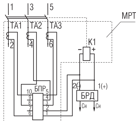
Стационарное исполнение
