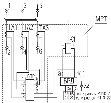
Выдвижное исполнение
