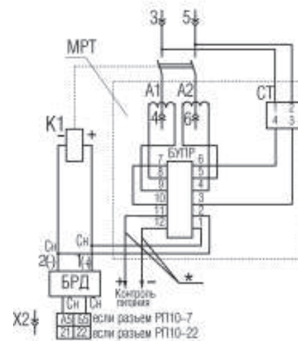
Выдвижное исполнение
