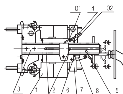
Рисунок 9 - Установка ручного привода
