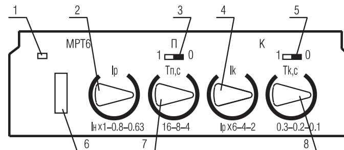
Рисунок 13 - Общий вид лицевой панели блока MPT2
