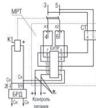
Стационарное исполнение
