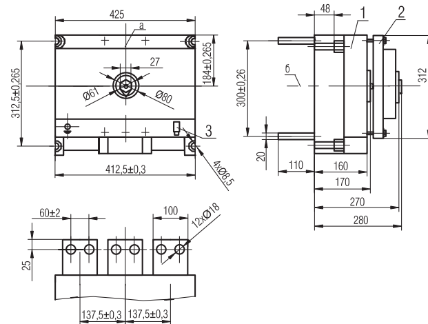
Масса - не более 56 кг; 1 - выключатель, см. рисунок 1; 2 - привод электромагнитный; 3 - соединитель цепи управления электромагнитного привода а - горизонтальная ось электромагнитного привода. Рисунок 4 - Выключатели стационарного исполнения с задним присоединением на номинальный ток 1600 А с электромагнитным приводом
