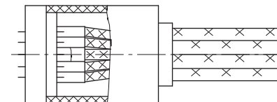
Вилка соединительная. Провода припаиваются потребителем.
