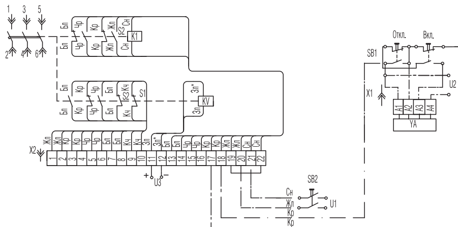
Рисунок 3 - Схема электрическая принципиальная выключателей выдвигного исполнения с дополнительными сборочными единицами
