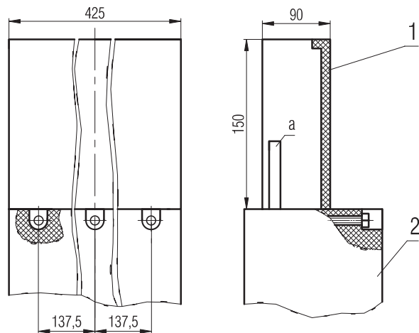
1 - козырек; 2 - выключатель а - вывод выключателя для присоединения шины Рисунок 4 - Установка козырька на выключатель с передним присоединением внешних проводников
