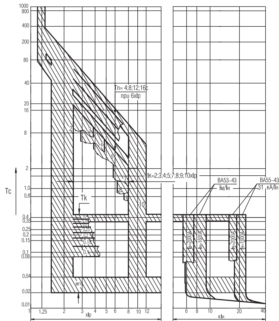
Рисунок 1 - Время-токовая характеристика выключателей переменного тока ВА53-43 и ВА 55-43 с блоками МРТ1, МРТ2;
