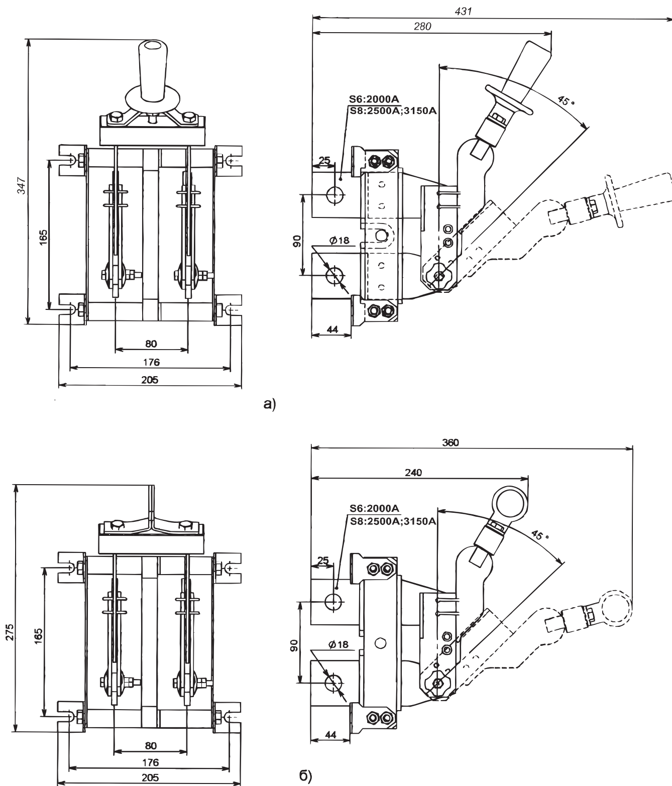
Рис. 42. Разъединитель PE19 однополюсный, заднего присоединения шин а) PE19-44(45; 46)-12210-00 УХЛ3 с центральной рукояткой; б) PE19-44(45; 46)-12290-00 УХЛ3 с центральной штангой
