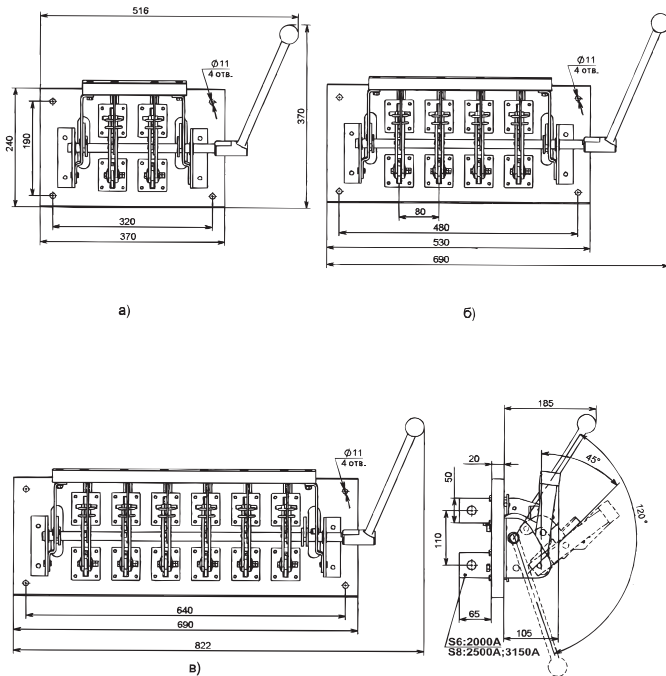
Рис. 48. Разъединитель PE19 с боковой рукояткой, заднего присоединения шин а) PE19-44(45; 46)-12220-00 УХЛЗ; б) PE19-44(45; 46)-22220-00 УХЛЗ; в) PE19-44(45; 46)-32220-00 УХЛЗ
