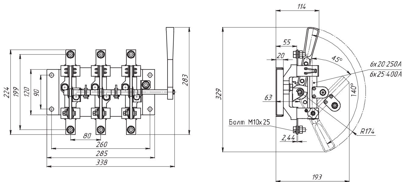
Рис. 6. Разъединитель РЕ19-35(37)-31120-00 УХЛЗ с боковой рукояткой
