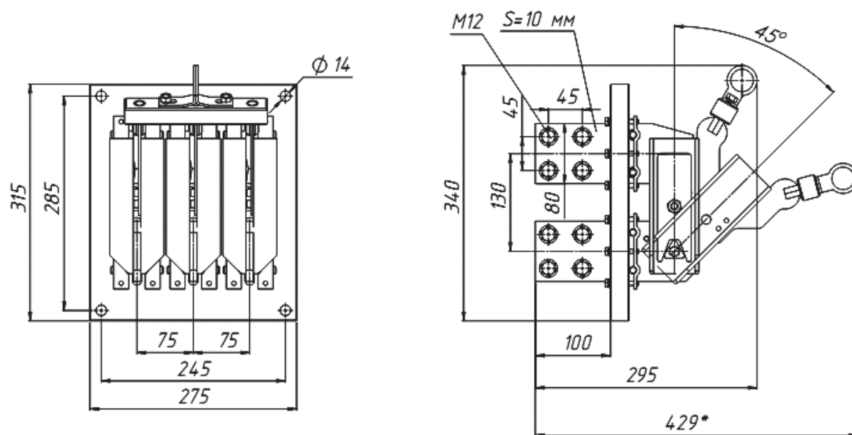
Рис. 51. Разъединитель PE19 с рычагом для полюсного оперирования штангой PE19-49-12290-00 УХЛ3
