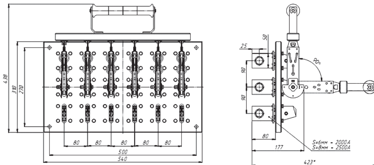
Рис. 50. Разъединитель PE19 на два направления с центральной рукояткой PE 19-44 (45; 46)-72210-00 УХЛ3
