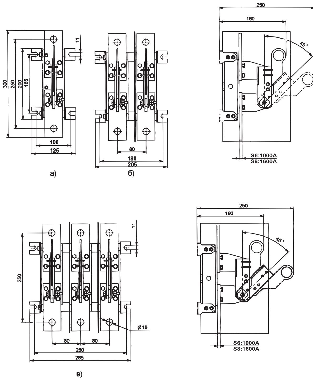
Рис. 19. Разъединитель PE19 с рычагом для полюсного оперирования штангой а) PE19-41(43)-11160-00 УХЛ3; б) PE19-41(43)-21160-00 УХЛ3; в) PE19-41(43)-31160-00 УХЛ3
