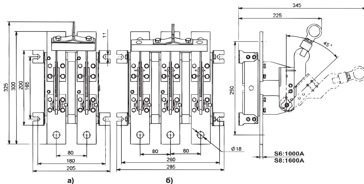
Рис. 27. Разъединитель PE19 с центральной штангой а) PE19-41(43)-21190-00 УХЛЗ; б) PE19-41(43)-31190-00 УХЛЗ
