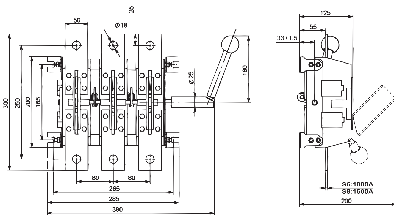
Рис. 17. Разъединитель РЕ19-41(43)-31150-00 УХЛЗ с боковой смещенной рукояткой
