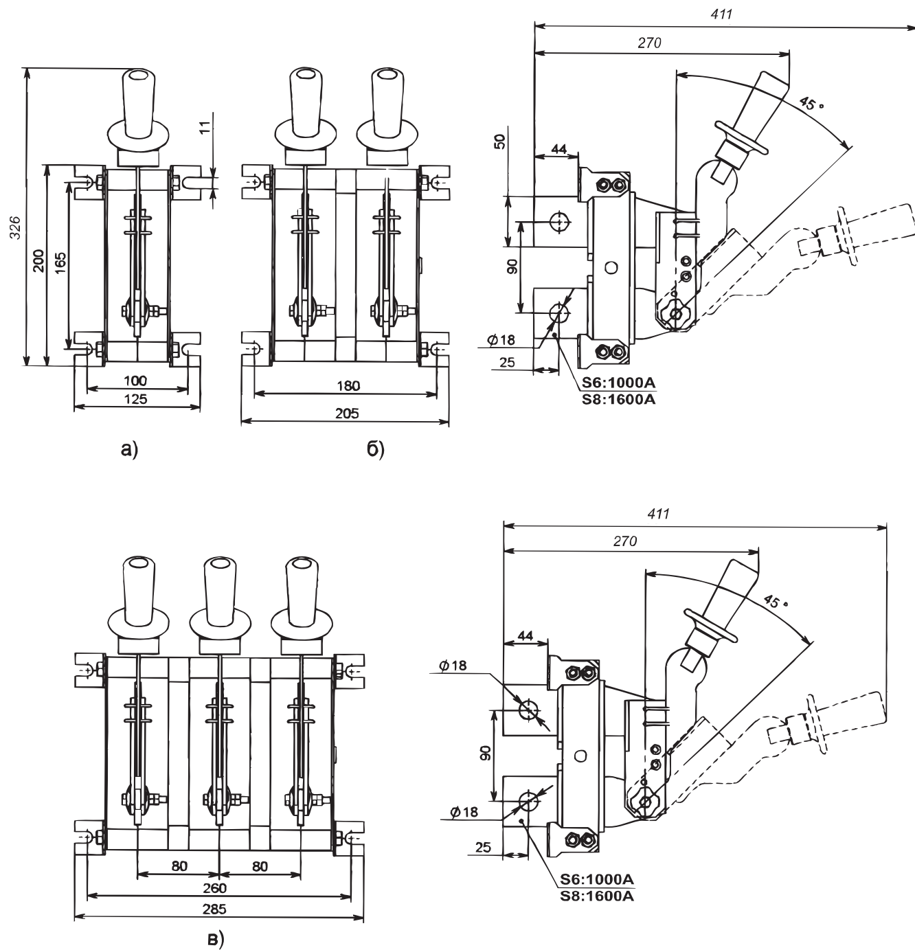
Рис. 24. Разъединитель PE19 с рукояткой для полюсного оперирования, заднего присоединения шин а) PE19-41(43)-12270-00 УХЛЗ; б) PE19-41(43)-22270-00 УХЛЗ; в) PE19-41(43)-32270-00 УХЛЗ
