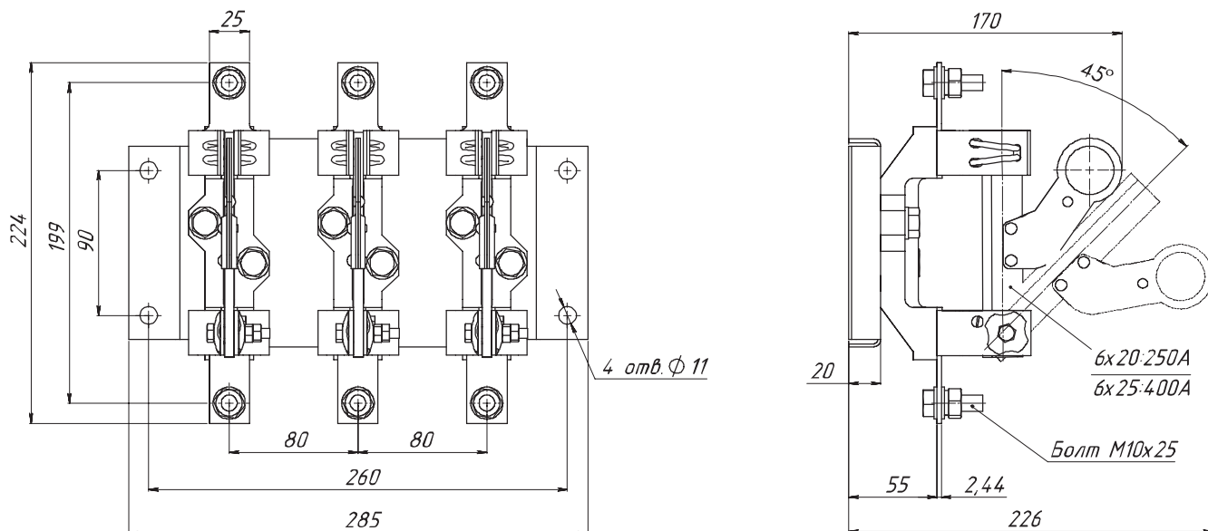
Рис. 5. Разъединитель РЕ19-35(37)-31160-00 УХЛЗ с рычагом для полюсного оперирования штангой
