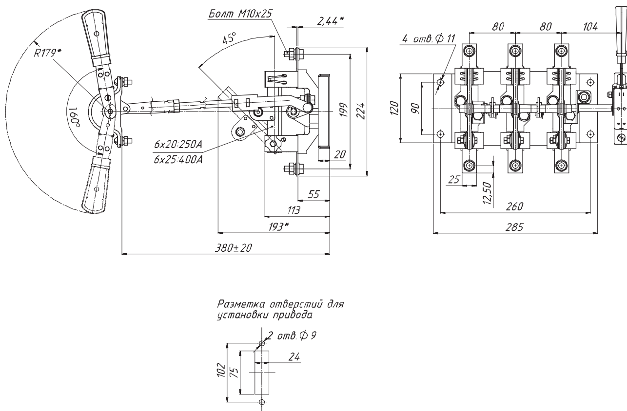
Рис. 7. Разъединитель PE19-35(37)-31140-00 УХЛ3 с передней смещенной рукояткой
