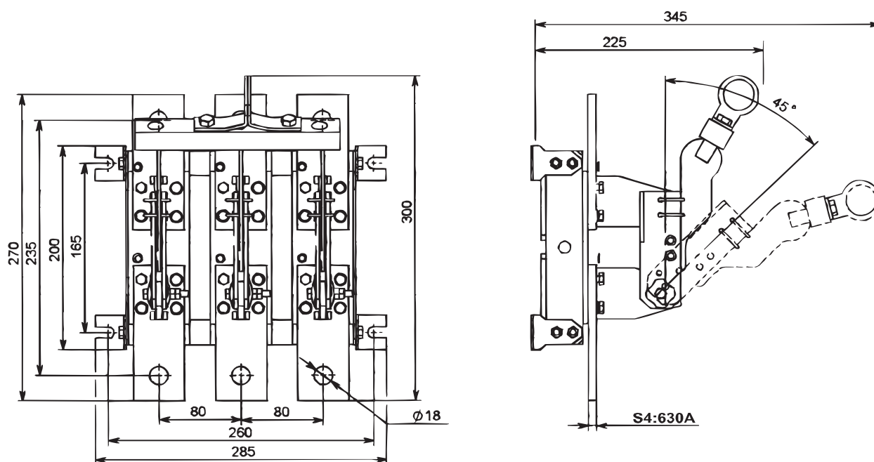
Рис. 8. Разъединитель PE19-39-31190-00 УХЛ3 с центральной штангой
