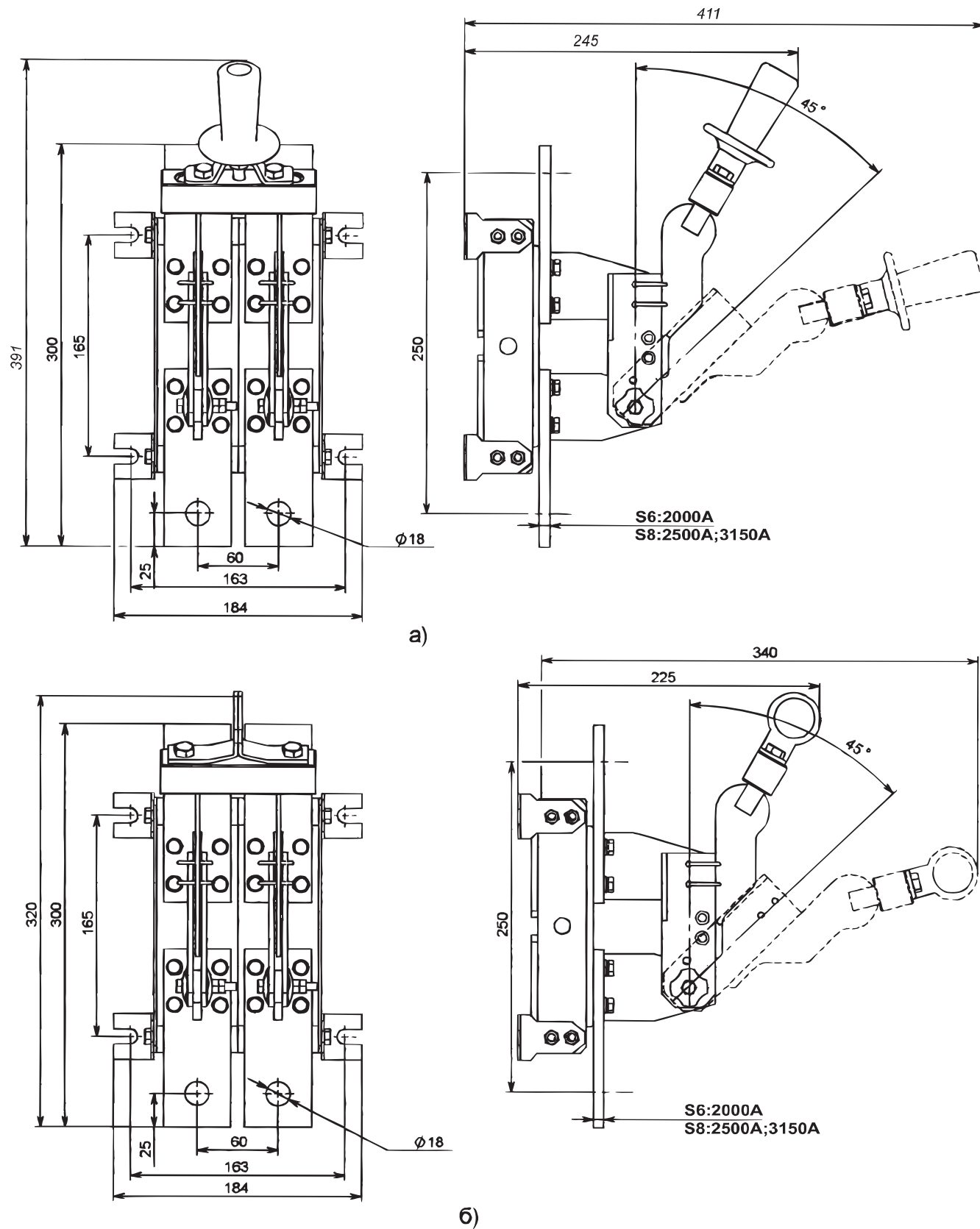
Рис. 41. Разъединитель PE19 однополюсный а) PE19-44(45; 46)-11110-00 УХЛЗ с центральной рукояткой; б) PE19-44(45; 46)-11190-00 УХЛЗ с центральной штангой
