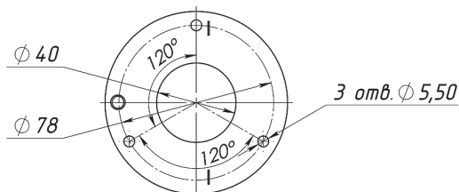
Рис. 40. Разъединитель РЕ19-41(43)-72250-00 УХЛЗ на два направления с боковой смещенной рукояткой
