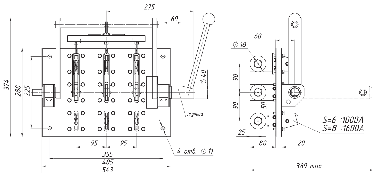
Рис. 39. Разъединитель РЕ19-41(43)-72220-00 УХЛЗ на два направления с боковой рукояткой
