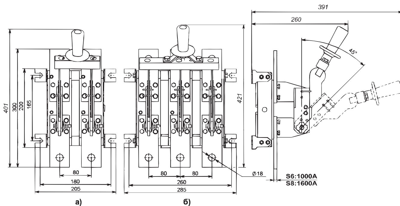
Рис. 28. Разъединитель PE19 с центральной рукояткой а) PE19-41(43)-21110-00 УХЛЗ; б) PE19-41(43)-31110-00 УХЛЗ
