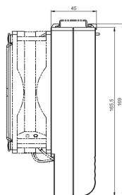
Крепление винтами
